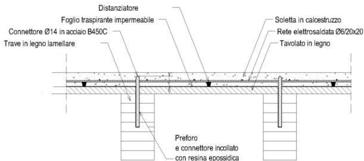
Figura 1: sezione tipo di un solaio misto legno-calcestruzzo
